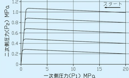
YR-70 圧力変動曲線
