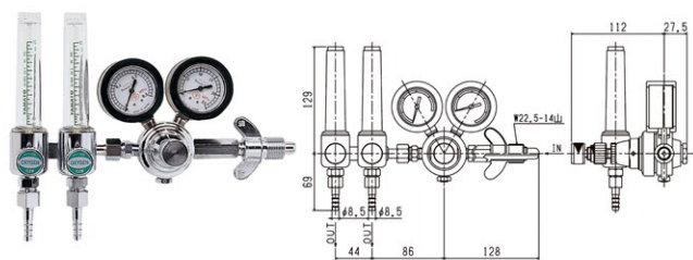
YR-90KW-F2M-10 (流量計2連式)
