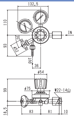
出口ストップバルブ付
