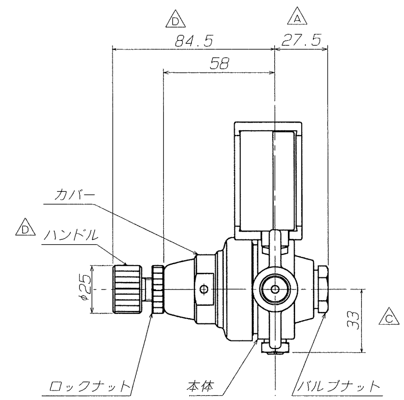
A矢視 (尺度 1:2)
