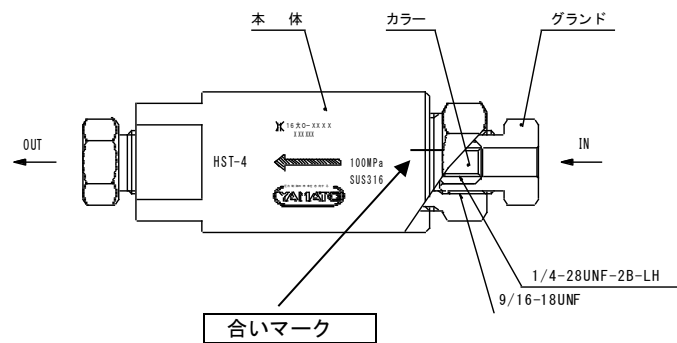
超高压ストレーナ HST-4
