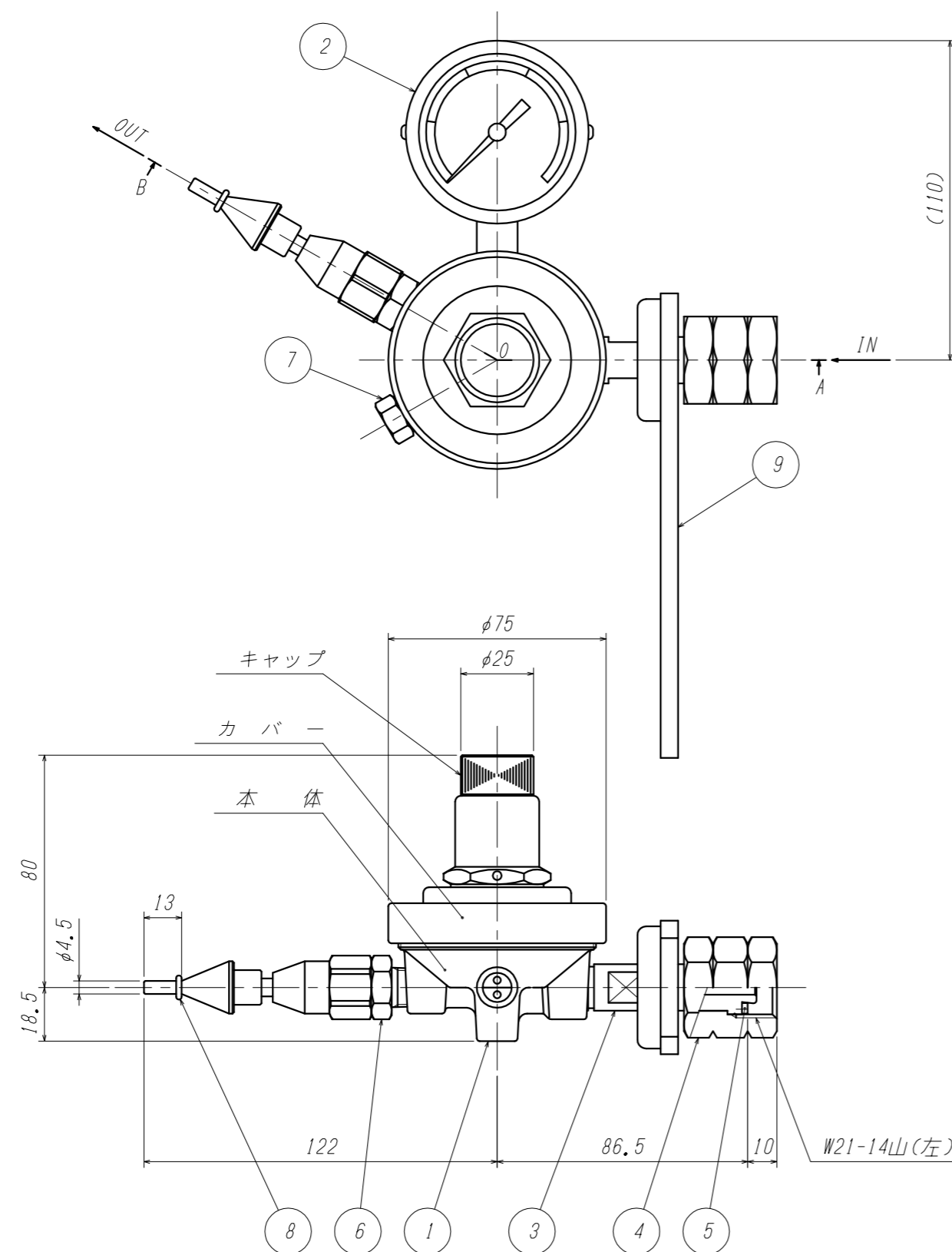
B-0-A矢視
