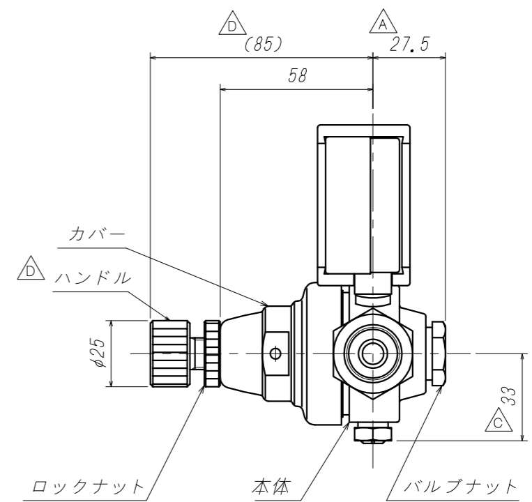
A矢視(尺度 1:2)
