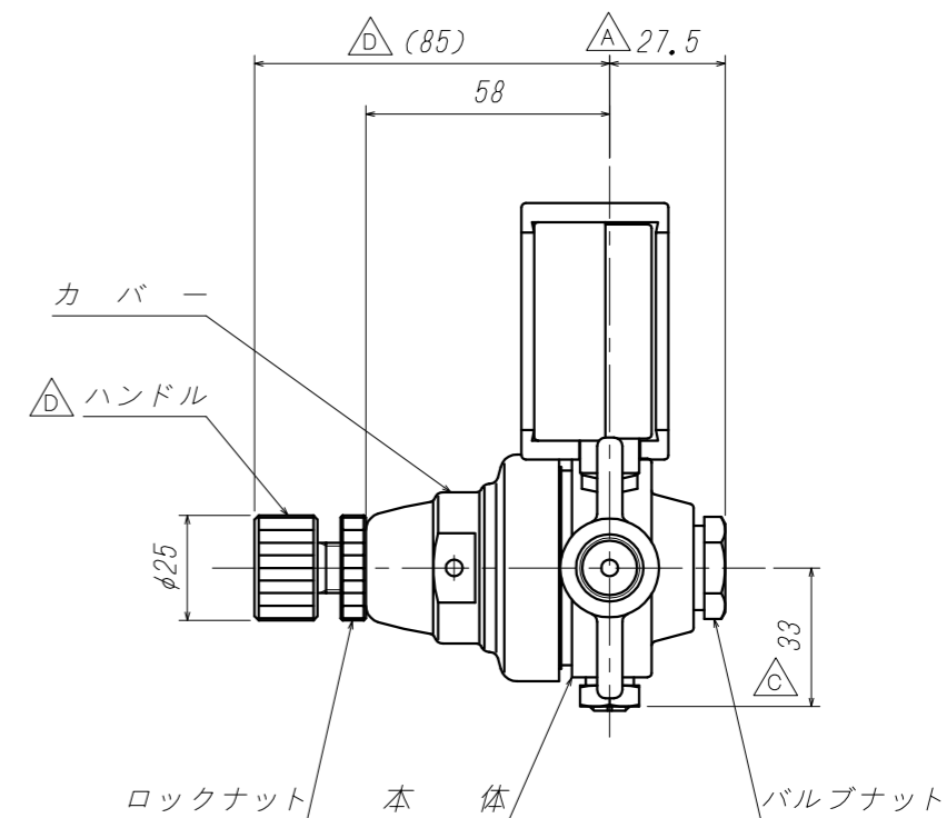
A矢視(尺度 1:2)
