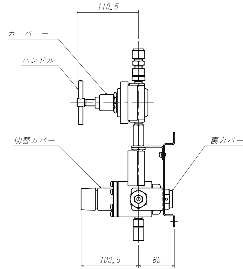
C矢視(縮尺 1:4)
