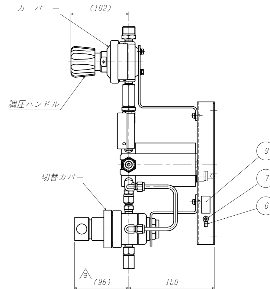
A矢視 (尺度1:4)
