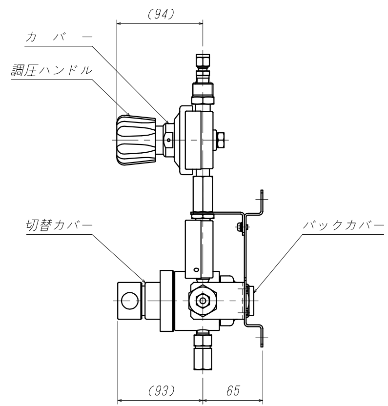
側面図(縮尺 1:4)
