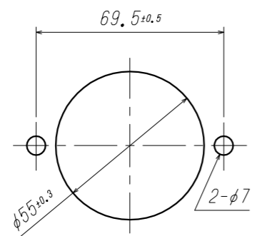
パネルマウント加工寸法
