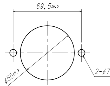
パネルマウント加工寸法
