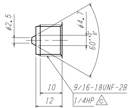
1/4HP 詳細図 (Scale:1) △B △C
