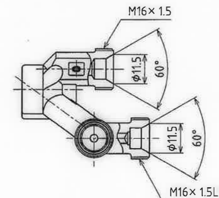
ホース継手接続部寸法
