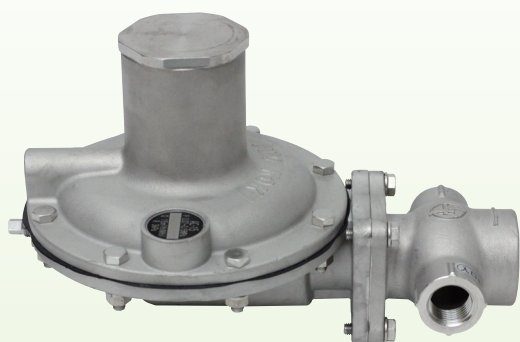
[ アンモニア用ガバナ ねじ込みタイプ ]
