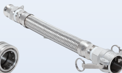
[ カムロックタイプ ]
