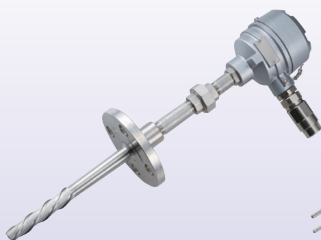
〔熱電対〕
