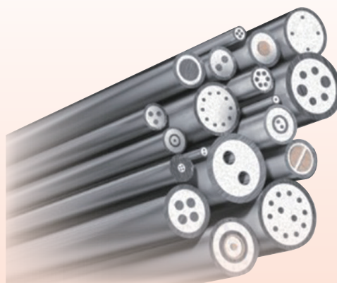
〔MIケーブル〕
