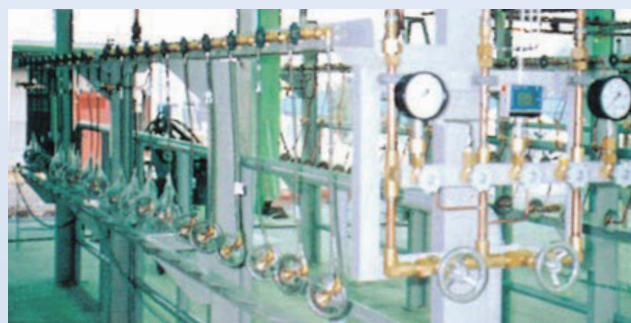
[ 充填架台 ]
