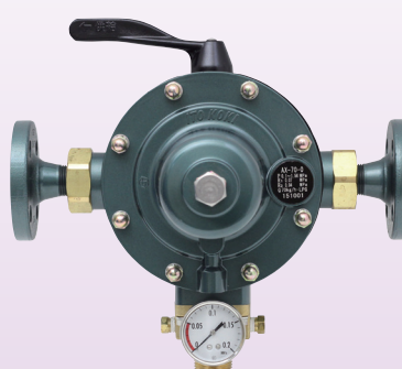
[ 自動切替 大流量タイプ ]
