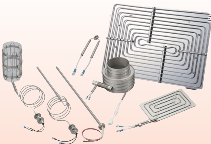
〔マイクロヒーター〕
