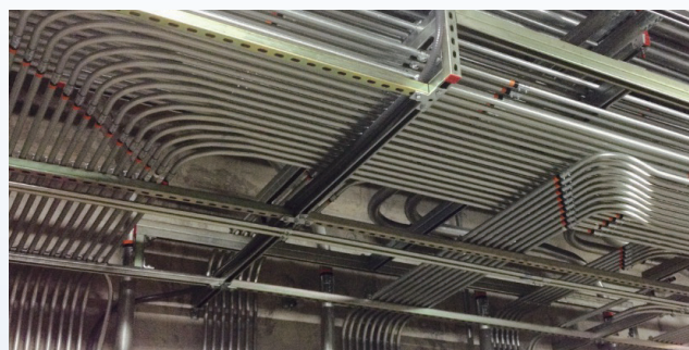
[ 集中配管 ]
