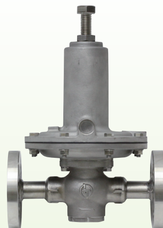
[ アンモニア用レギュレータ フランジタイプ ]
