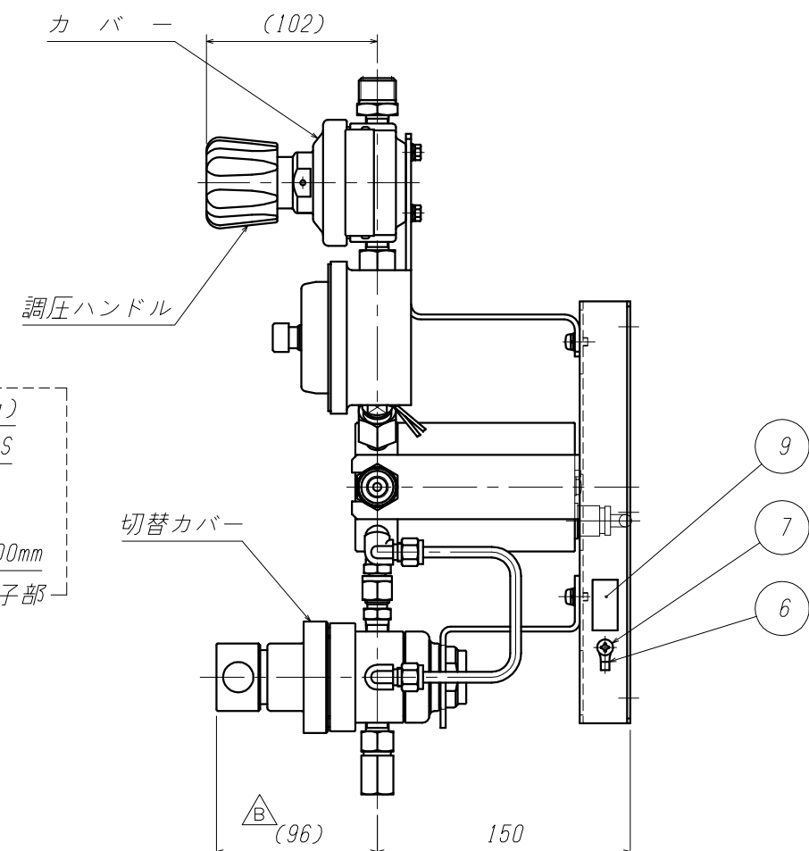
A矢視 (尺度1:4)
