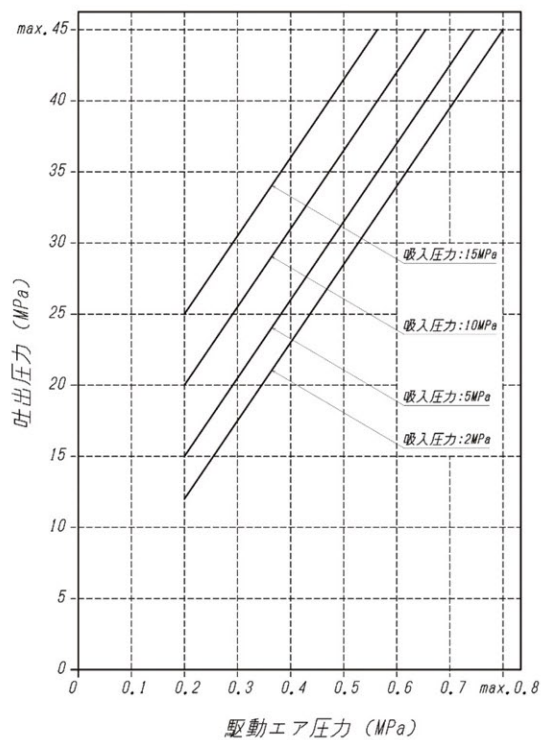
吐出圧力と駆動エア圧力の関係図
