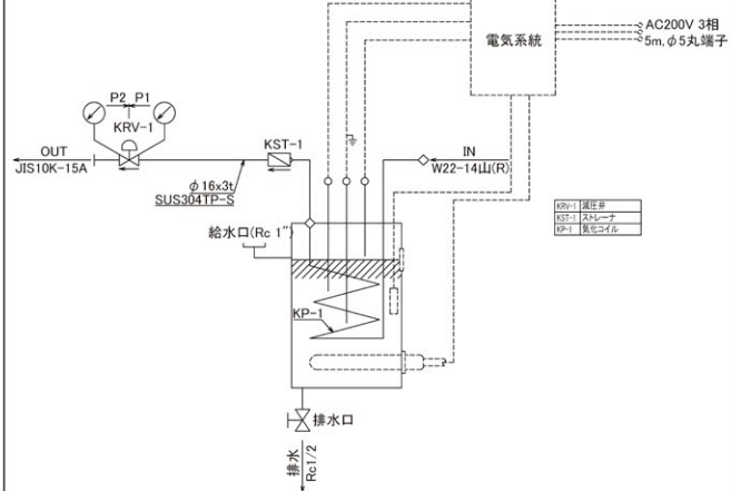
フロー図
