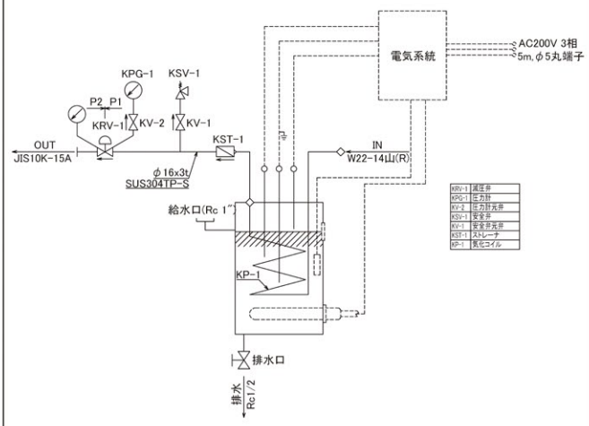
フロー図
